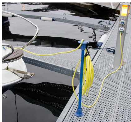
Kabelholder med elkabel fra strømsøyle til båt
